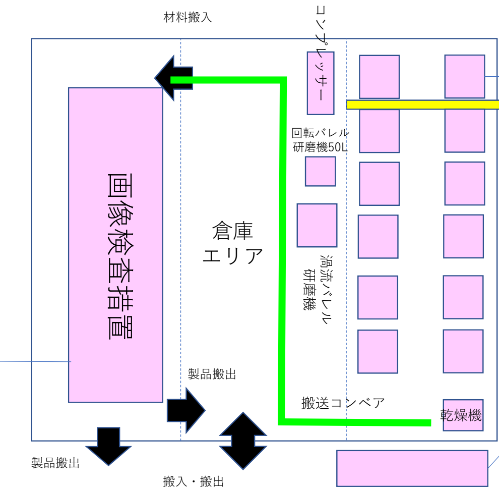
回転バレル研磨機100L × 12機
